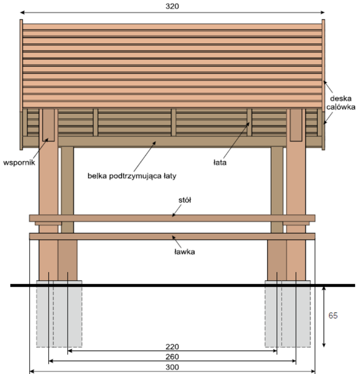
schemat wiaty z przodu
